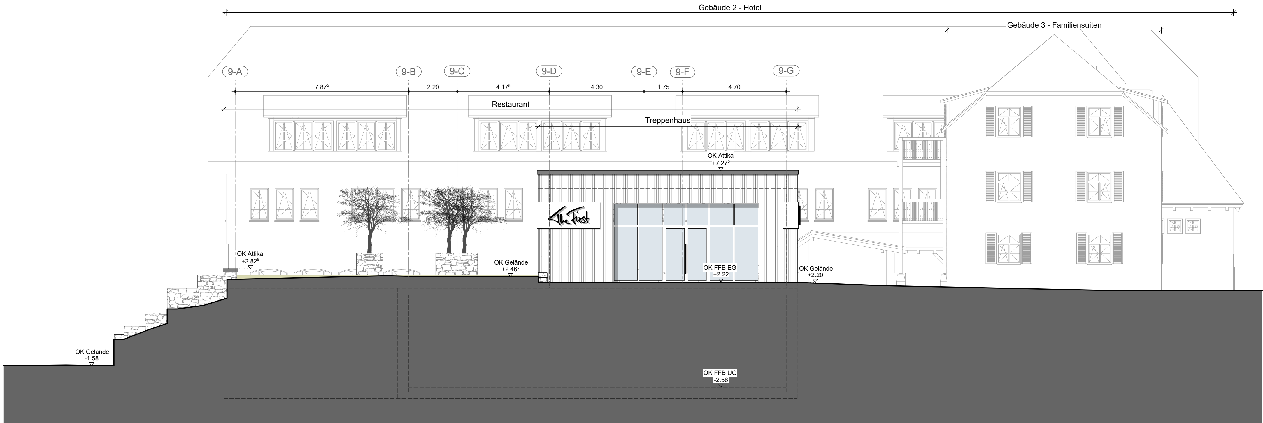
Ansicht Südwest
