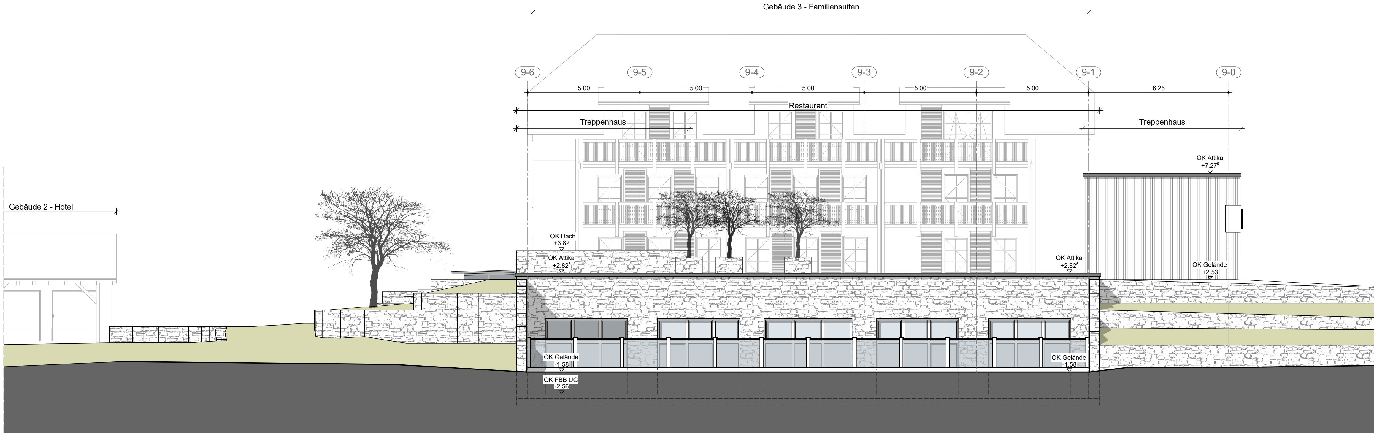
Ansicht Nordwest
